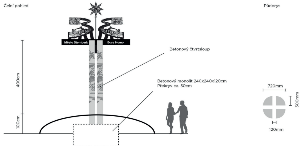
Čelní pohled
